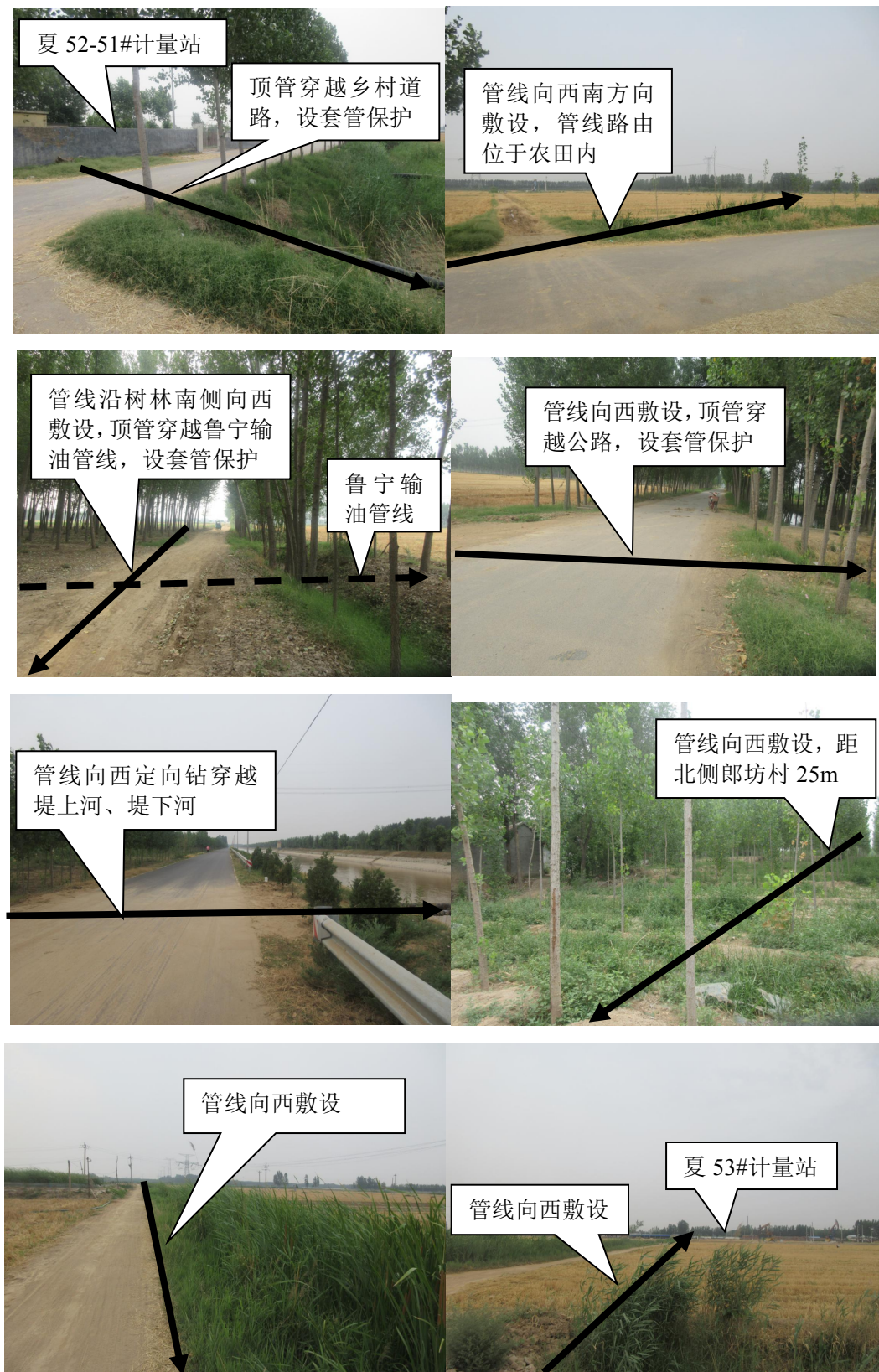
图 5.2-2 夏 53 站至夏 52-51 站外输管线现场示意图
