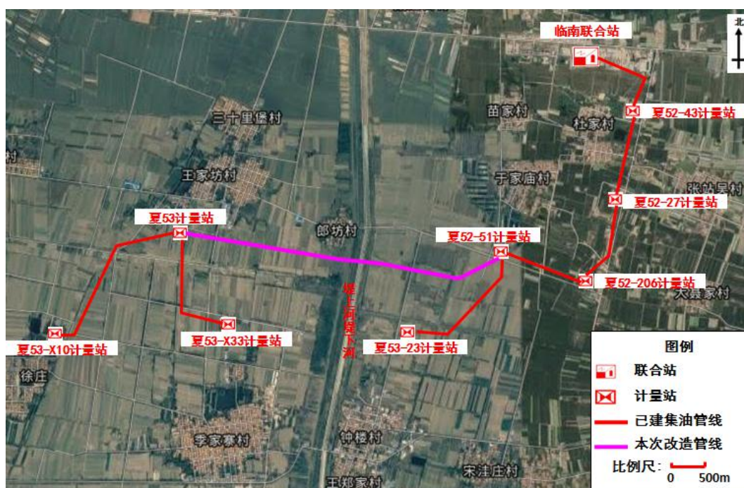
图 2.3-2 夏 53 站至夏 52-51 站混输管线及周边外输管线示意图
