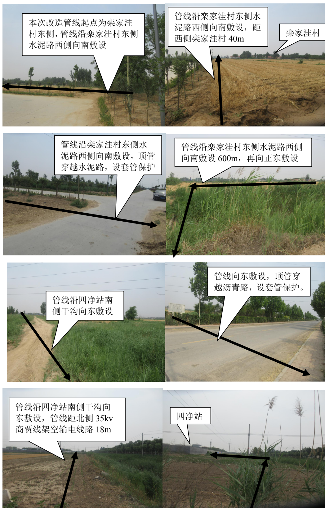
图 5.2-1 商 8-17 阀组至四净站外输管线现场示意图
