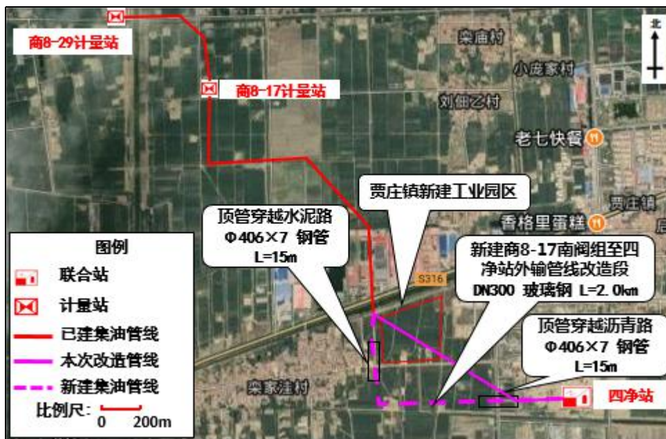
图 2.4-1 商 8-17 站南阀组至四净站混输管线局部更换后走向示意图
